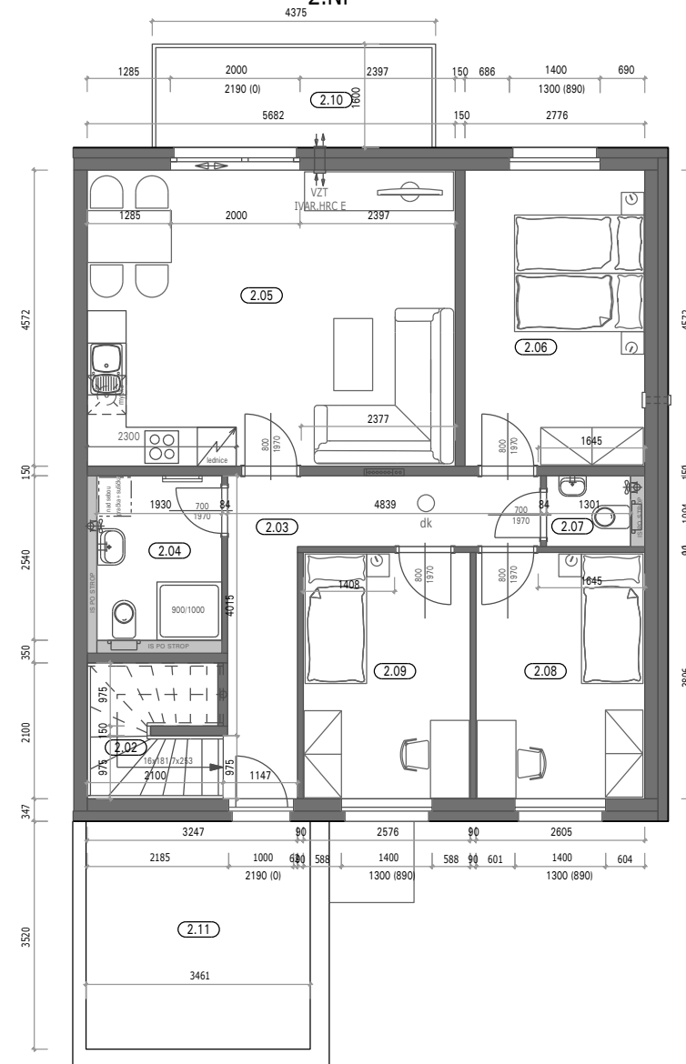
2.NP
