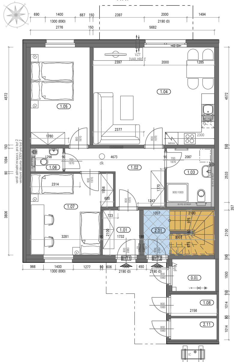
1.NP
